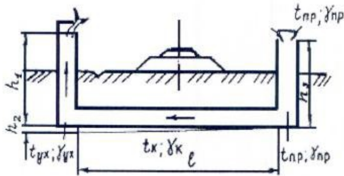
Рисунок Г.3 - Схема к аэродинамическому расчету системы вентиляции защитного кожуха Г.5.2 Потери давления на каждом расчетном участке
