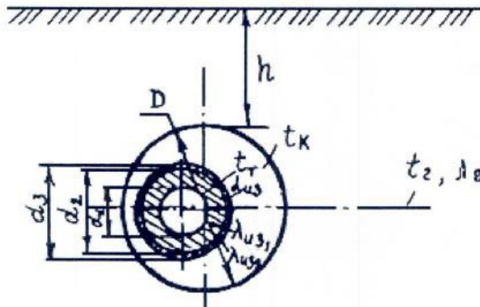
Рисунок Г.1 - Расчетная схема рабочего трубопровода в защитном футляре (кожухе) при пересечении земляного полотна
